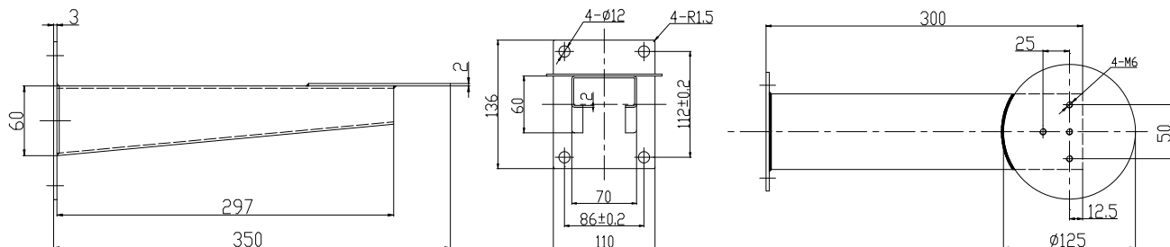
墙装支架尺寸
