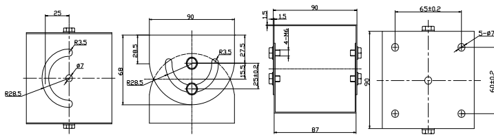
万向节支架尺寸
