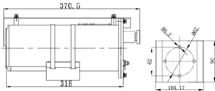
万向节支架尺寸
